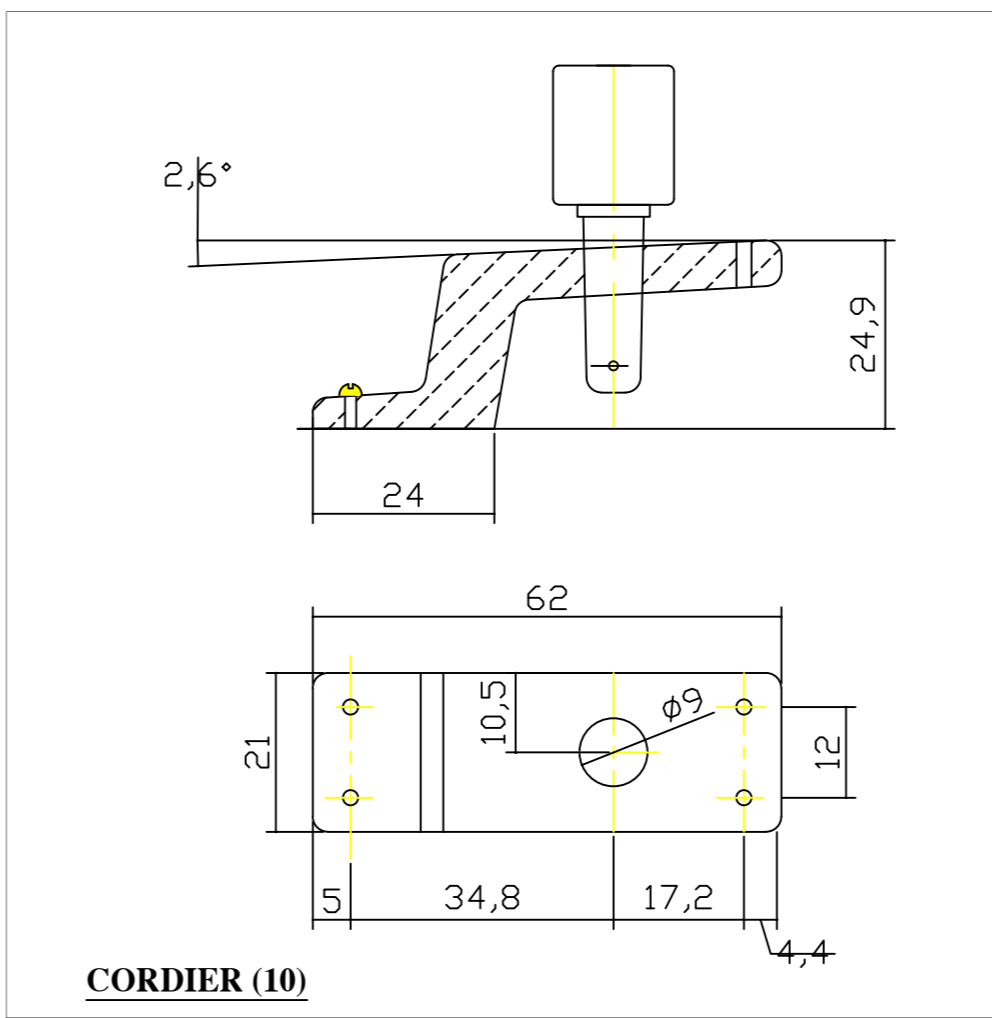
CORDIER (10)
